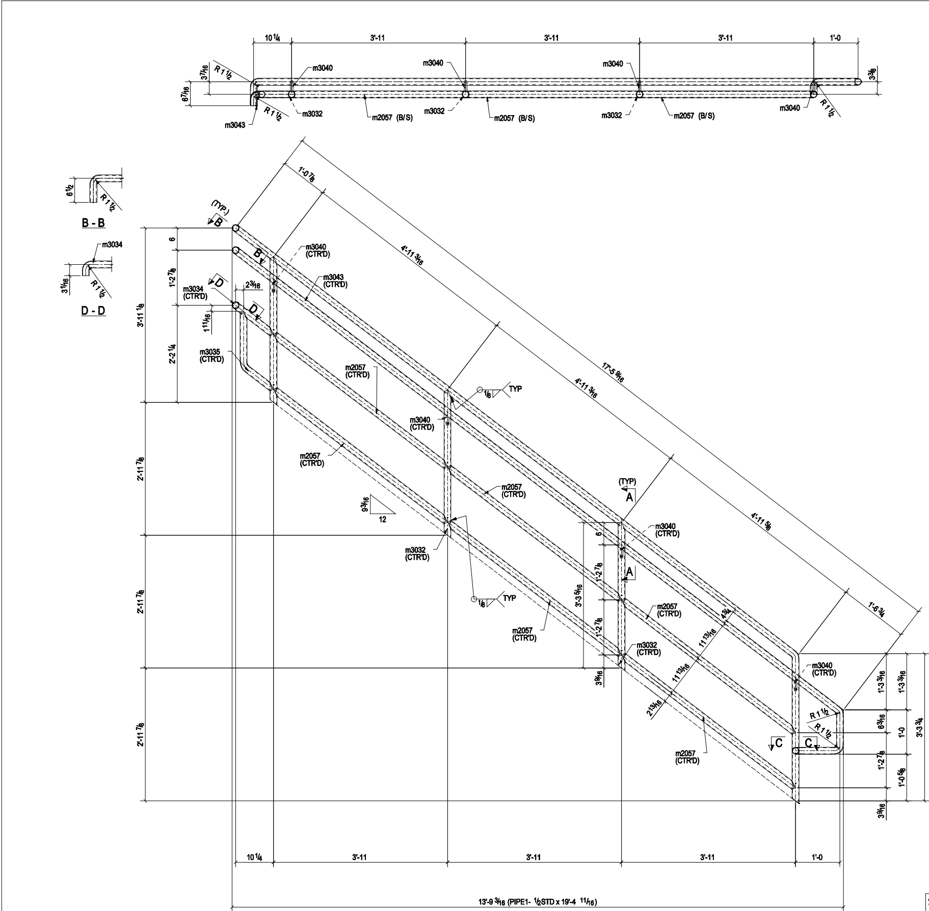
ONE - HANDRAIL - 3832A (GALV.)
